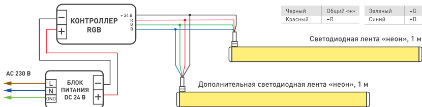
Схема 1. Подключение нескольких светодиодных лент «неон» с одной стороны. Арт. 047199
