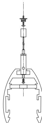
Рис. 3. Установка шинопровода на подвес
